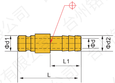
水咀 MB-STN
