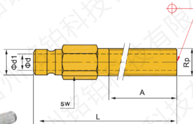
水咀 MB-EJP
