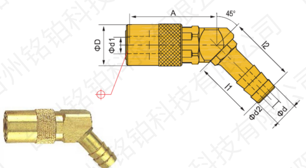
快速接头45° MB-SK(45°)
