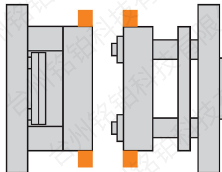
开模状态
