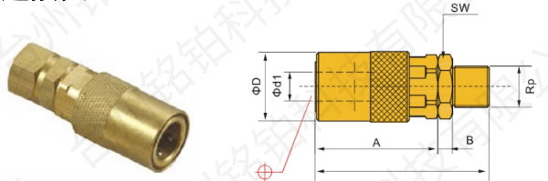
快速接头 MB-FSK
