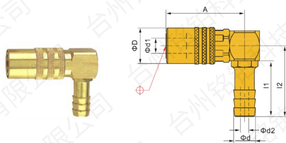
快速接头90° MB-SVK(90°)
