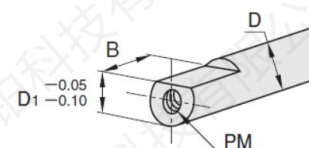
■适用斜推杆: 安装尺寸参考范例
