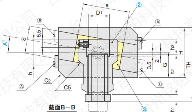
■适用斜推杆: 安装尺寸参考范例
