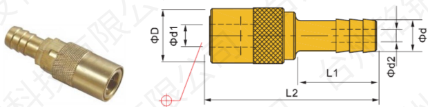
快速接头 MB-SK
