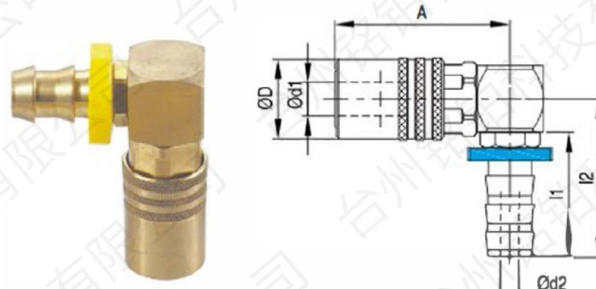
快速接头90°（封闭式） MB-JSL0214-SV
