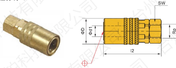
快速接头 MB-SVK-200
