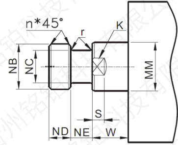
T:T型槽
