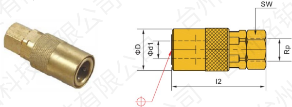
快速接头 MB-SK-200
