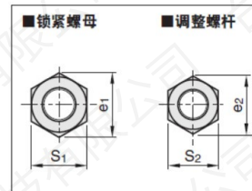
■适用斜推杆: 安装尺寸参考范例
