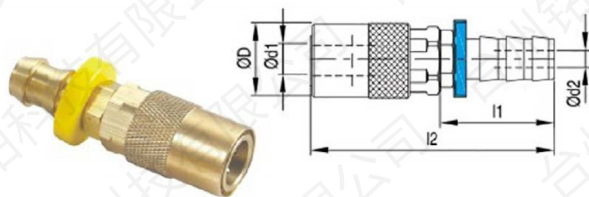
快速接头（开放式） MB-JSL0204
