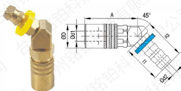
快速接头45°（封闭式） MB-JSL0224-SV
