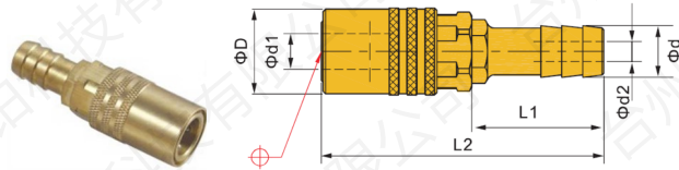
快速接头 MB-SVK
