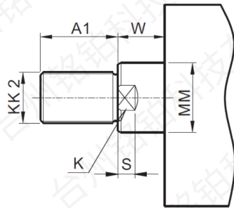
EX:外螺纹
