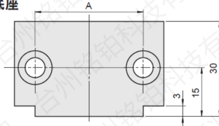
■底座
