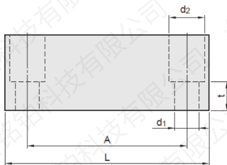
开模状态
