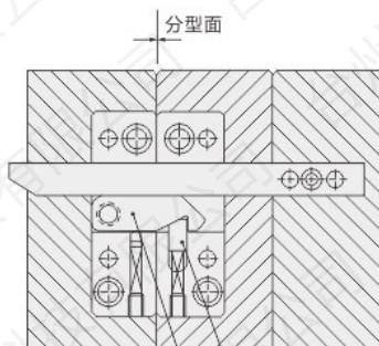
凸轮锁块 锁紧块 合模状态
