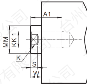
IN:内螺纹
