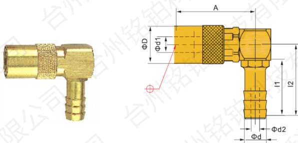
快速接头90° MB-SK(90°)
