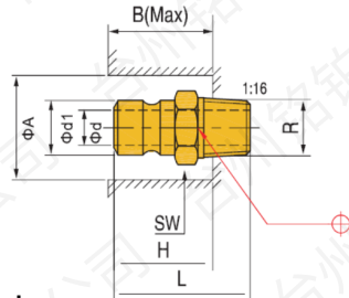
水咀（英制） MB-N
