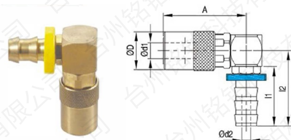
快速接头90°（开放式） MB-JSL0214
