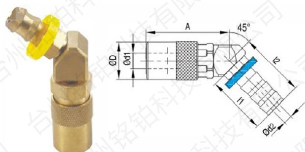
快速接头45°（开放式） MB-JSL0224
