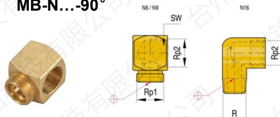
水咀 MB-N...-90°
