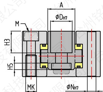
截面 B-B
