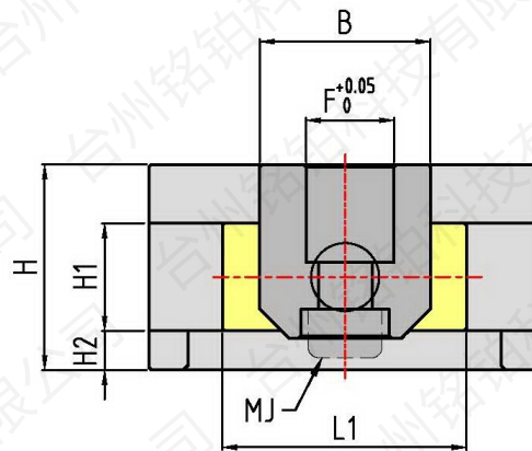
截面 A-A
