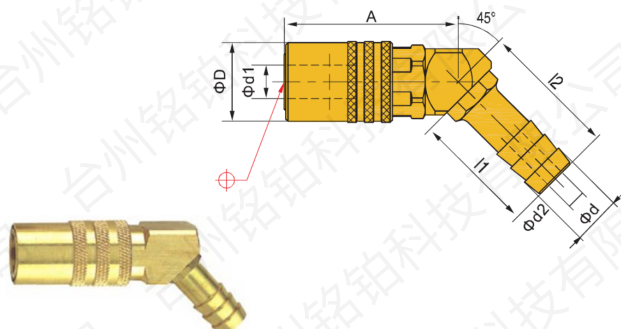
快速接头45° MB-SVK(45°)
